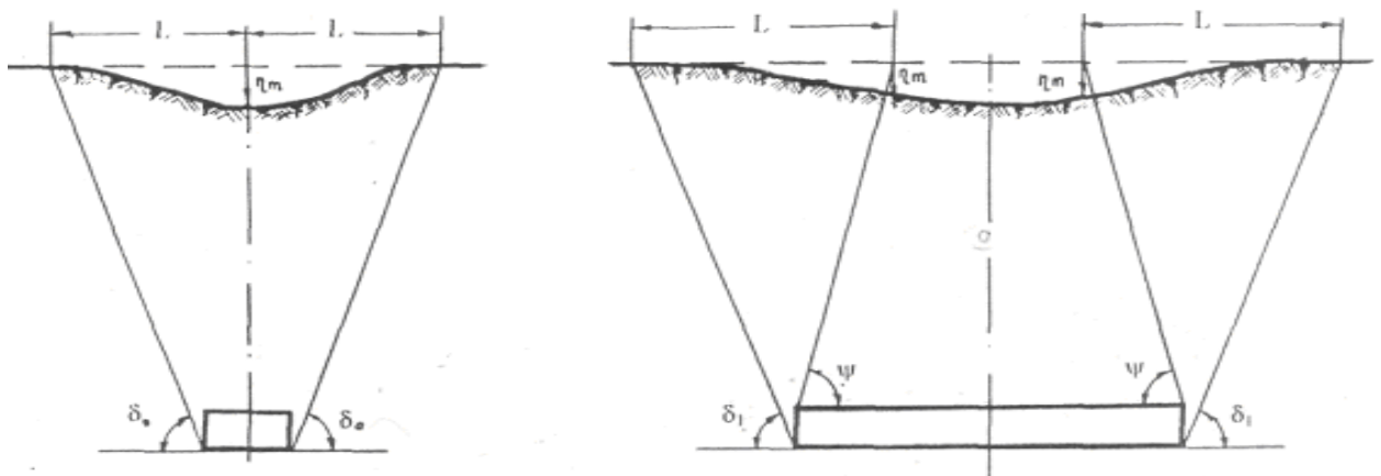
а) Разрез поперек объекта (неполная подработка)
